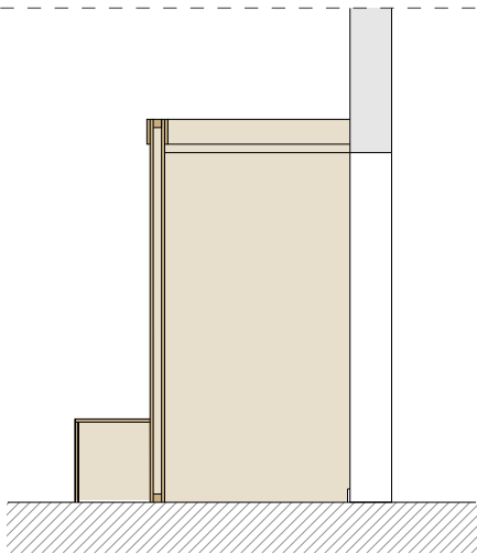
SEZ B-B'
